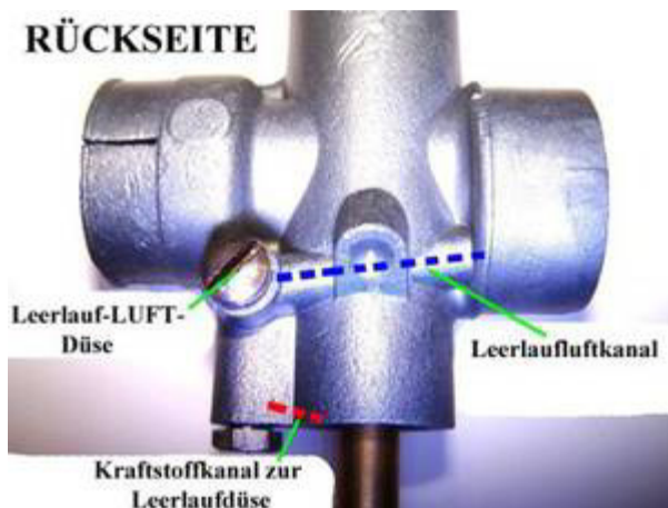
Bild 3 - Die Rückseite des Vergasers mit Leerlauf-LUFT-Düse
